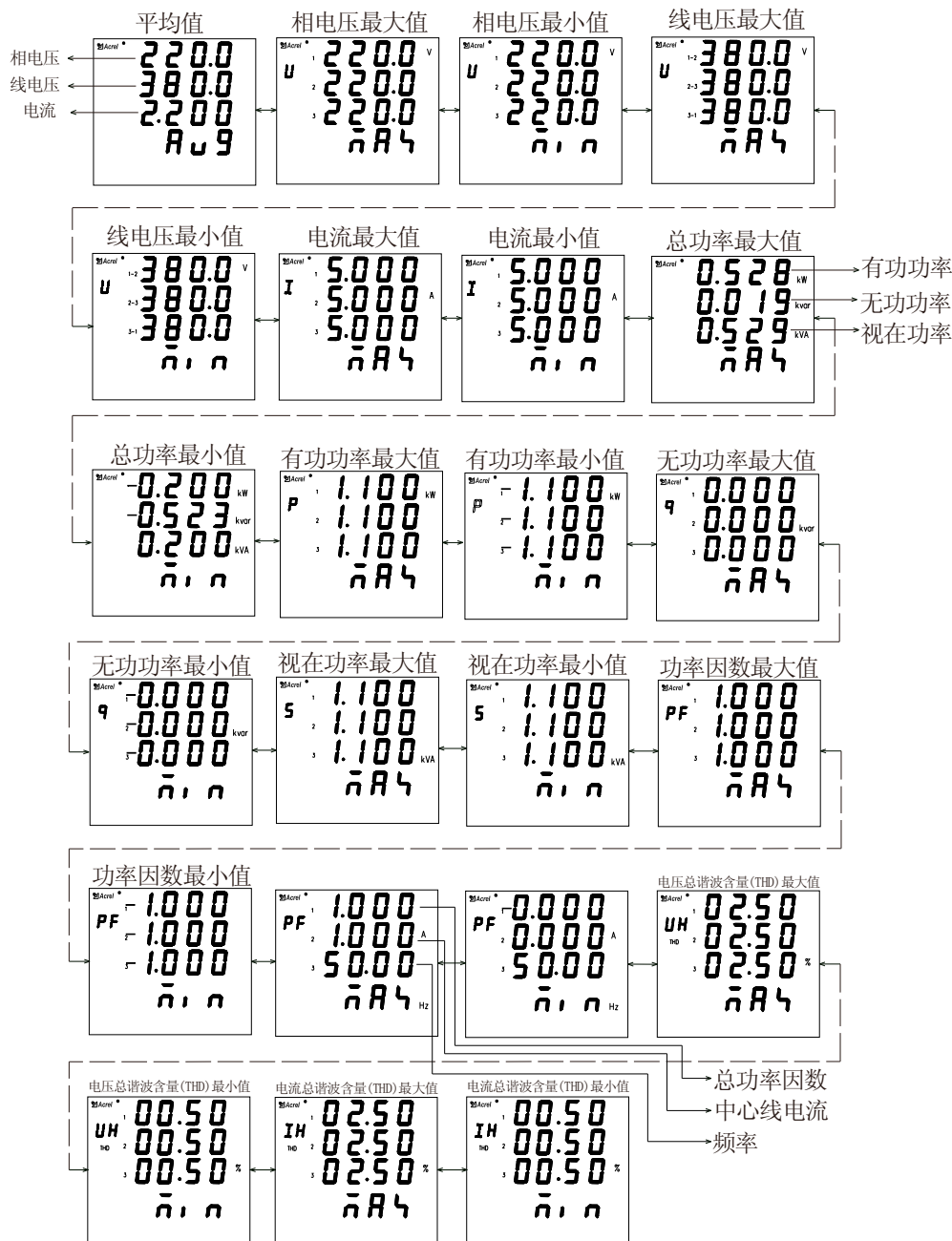
FUN1（功能）选项相关界面
